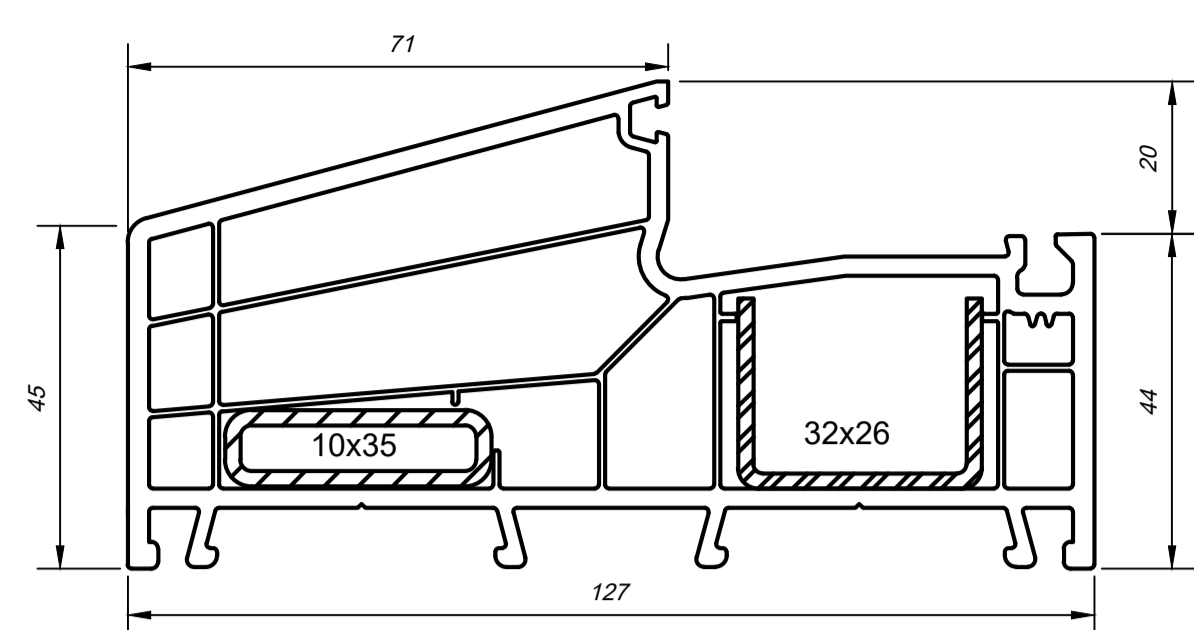
Рама широкая арт. 1727000
