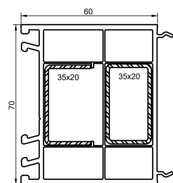
Расширитель 70x60мм арт. 8176 ( 629600 )
