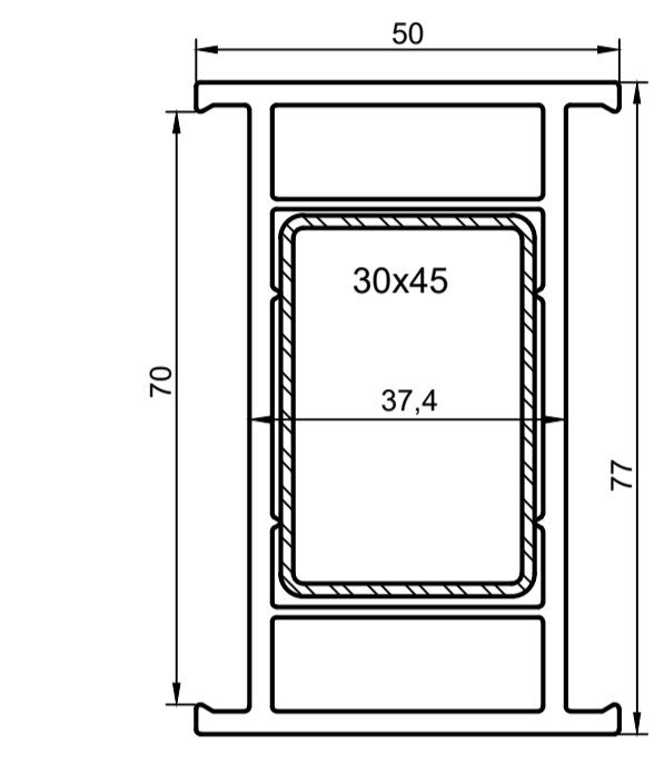
Соединитель (расширитель 70x37) арт. 8171 ( 111 )
