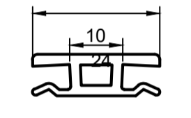
Профиль соединителя арт. 8083
