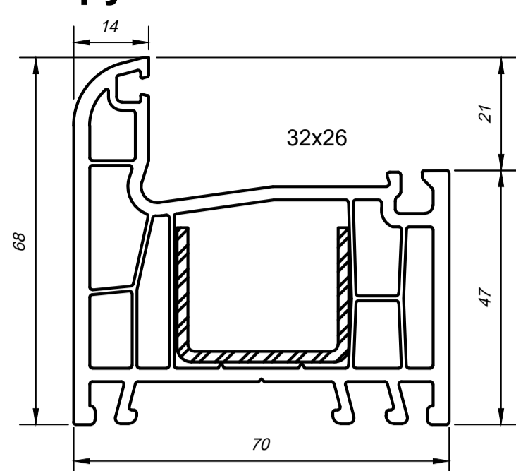
Рама арт. 1770000
