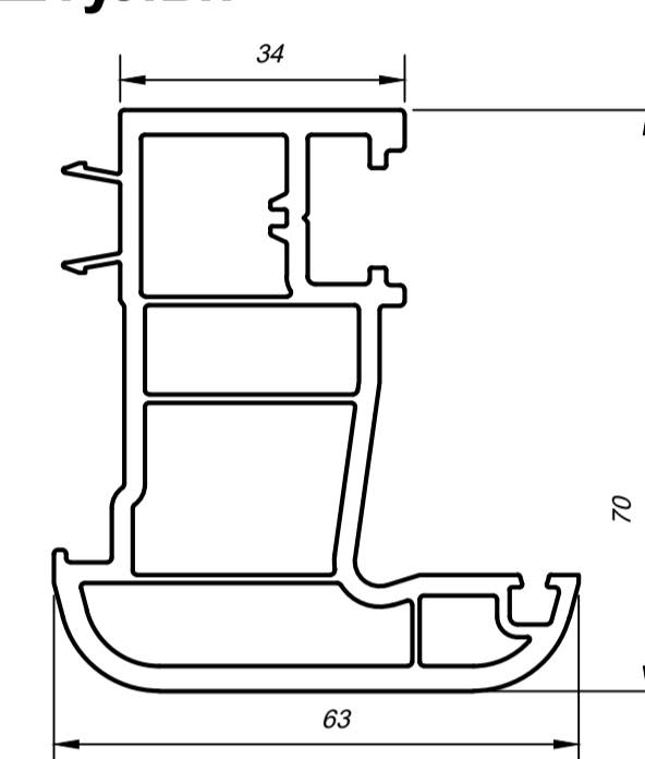
Штульп арт. 8160 ( 3763000 )
