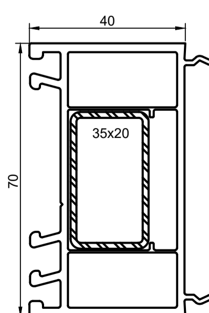
Расширитель 70x40мм арт. 8174 ( 629400 )
