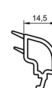
Штапик под с/п. 34 мм арт. 4214000
