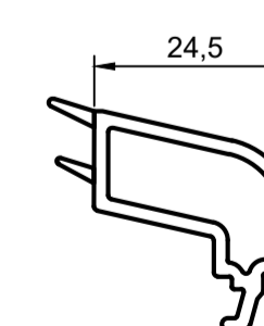
Штапик под с/п. 24мм арт. 4424000
