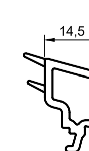
Штапик под с/п. 34 мм арт. 4114000
