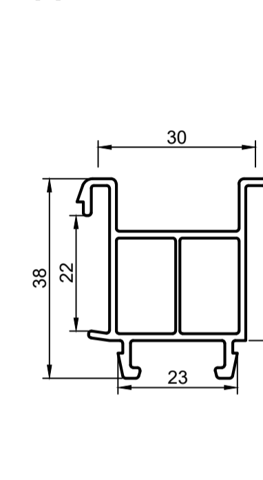
Подставочный арт. 112200 ( 201-1 )
