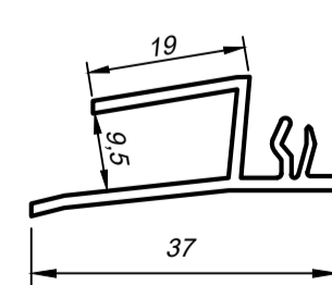
Стартовый арт. 630190
