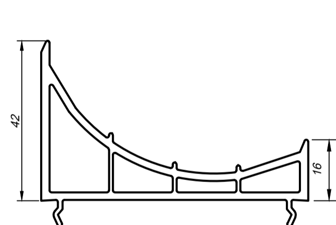
Адаптер эркера арт. 8182
