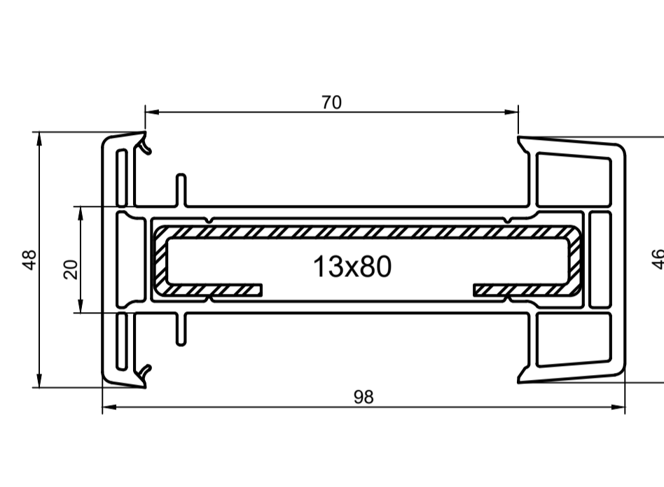
Статический усилитель арт. 8188 ( 118 )
