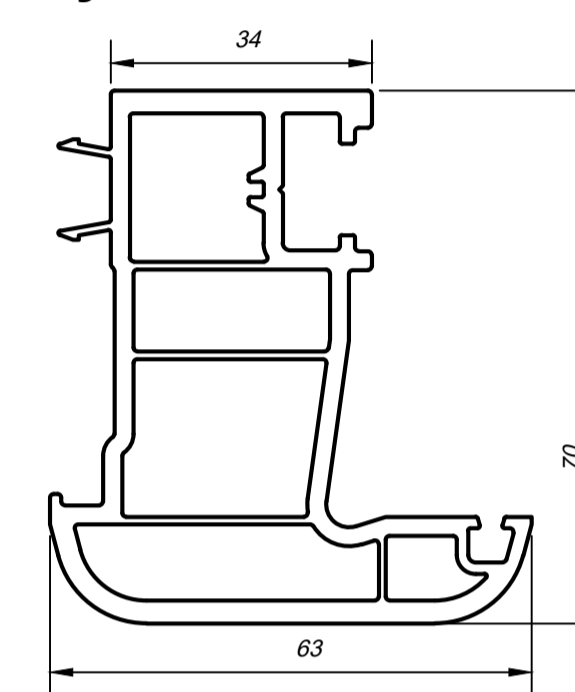
Штульп арт. 8160 ( 3763000 )
