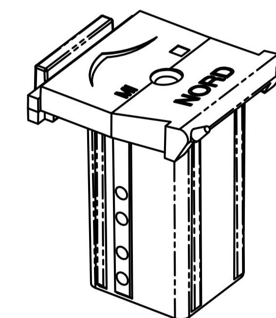
Соединитель импоста
