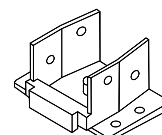
Соединитель импоста
