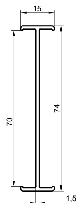
Соединитель 70 арт. 8189 ( 109 )
