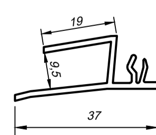
Стартовый арт. 630190
